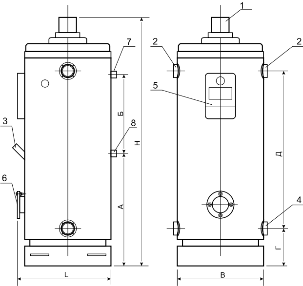
Рисунок 1. Внешний вид котла с ГВС 1 – Патрубок газохода 2 – Выходной патрубок системы отопления (подача) 3 – Смотровое отверстие 4 – Выходной патрубок системы отопления (обратка) 5 – Панель управления 6 – Патрубок для подсоединения горелочного устройства 7 – Патрубок для входа холодной воды на ГВС 8 – Патрубок для выхода горячей воды на ГВС
