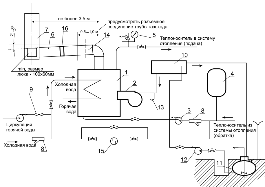
Рисунок 2. Схема обвязки котла с ГВС
