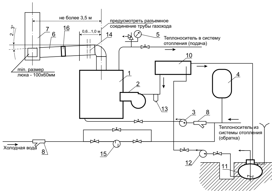
Рис.2 Схема обвязки котла без ГВС
